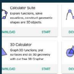
GeoGebra
